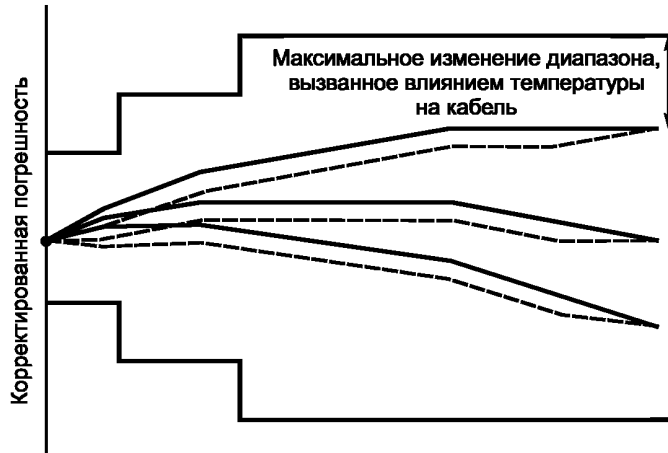
Рисунок 12 — Изменение диапазона из-за влияния температуры на кабель
